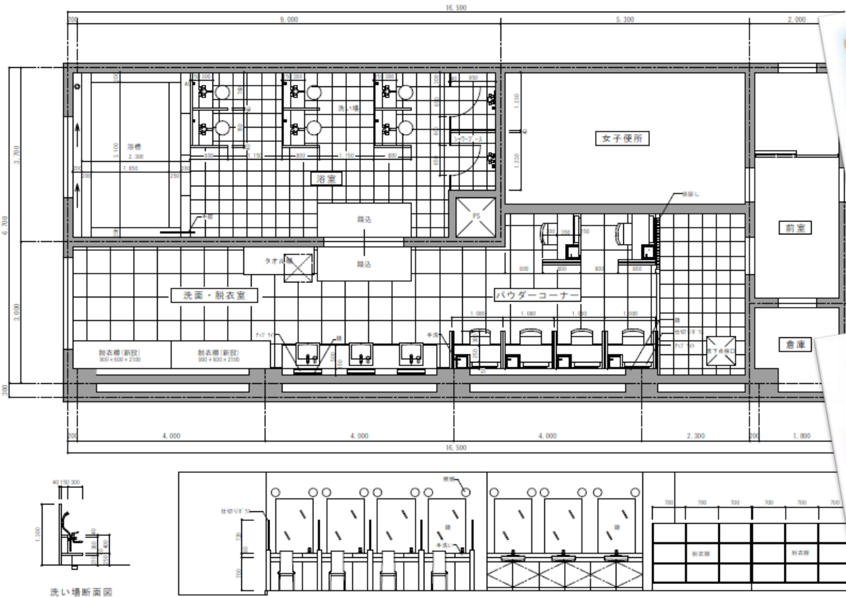
洗い場断面図
